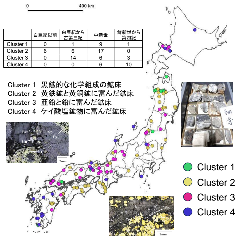
図1：日本列島全体にわたる熱水鉱床からの鉱石試料の化学成分濃度データに基づく4つのクラスターの分布、および各クラスターが各年代に何個あるかを表すクラスターと鉱床の形成年代との関係。各クラスターの特徴、鉱石の写真と顕微鏡画像の一例も表す。
