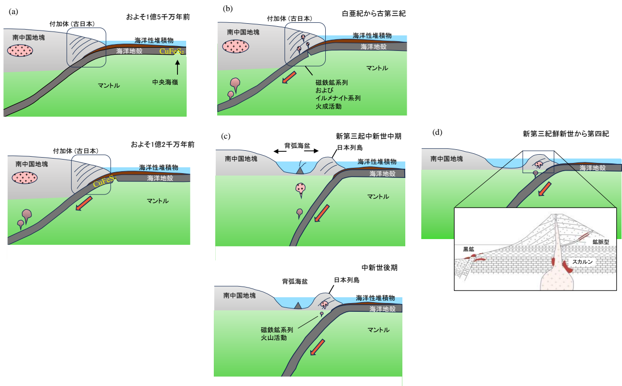
図2. 4つの地質年代(a)白亜紀以前、(b)白亜紀から古代三紀、(c)中新世、(d)鮮新世から第四紀における地殻変動場と鉱床生成プロセスのモデル図
