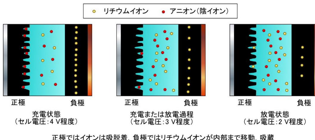
図1 リチウムイオンキャパシタの動作原理
